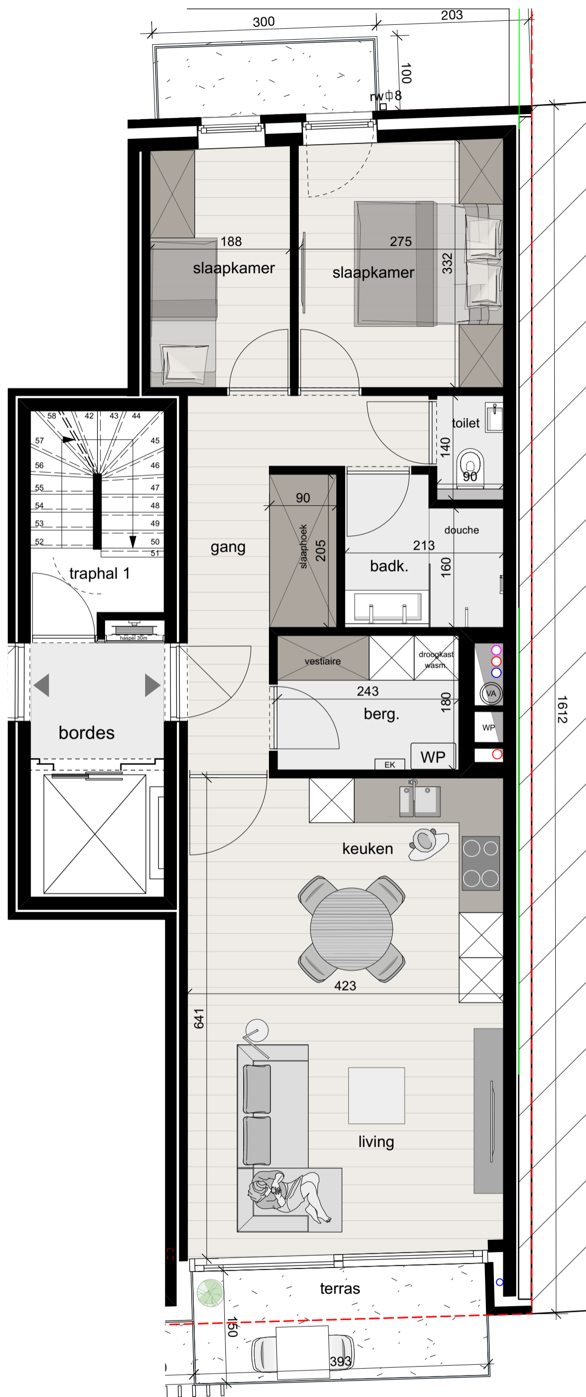
appartement 51/0302: bruto: 75 m 2 + 9 m 2 terrassen
